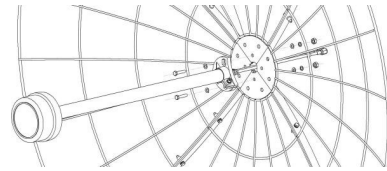
Шаг 2. Закрепите облучатель. 27 дБ
