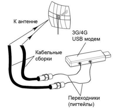
Пример подключения 3G/4G USB модема
