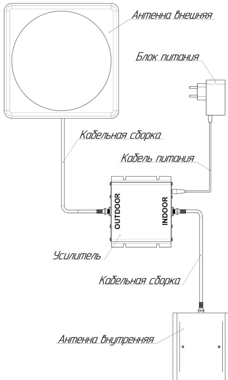
Схема 3 – Подключение комплекта
