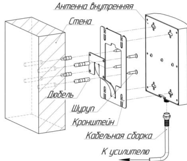
Схема 2. Монтаж внутренней антенны
