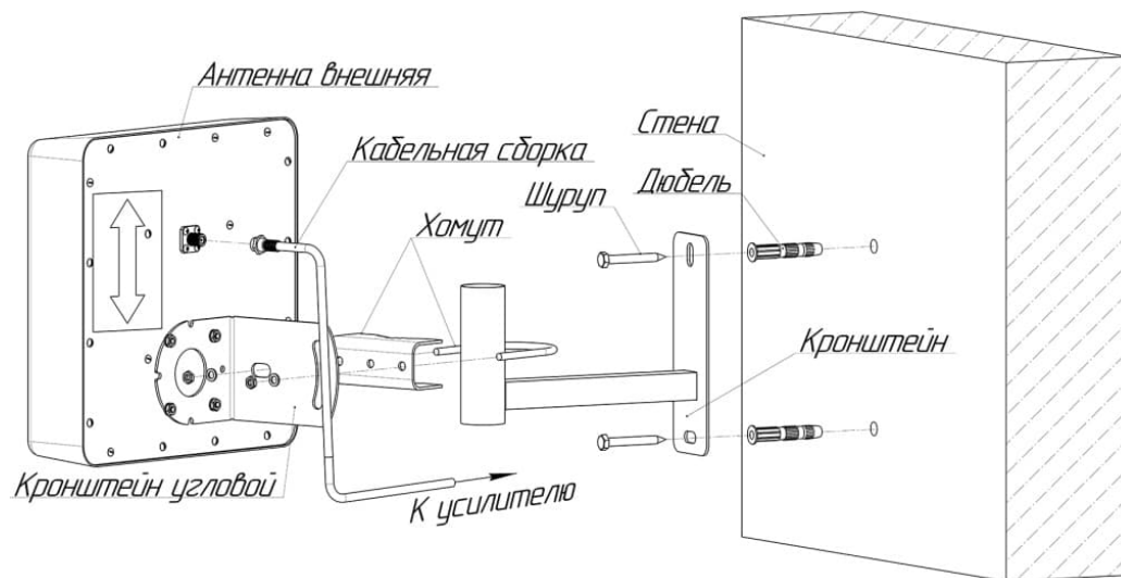
Схема 1 – Монтаж антенны на кронштейн КН-200
