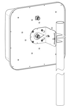
Монтаж антенны на мачте
