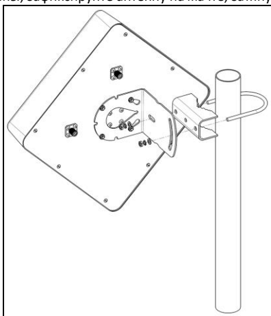
Рисунок 2 – монтаж антенны на мачте
