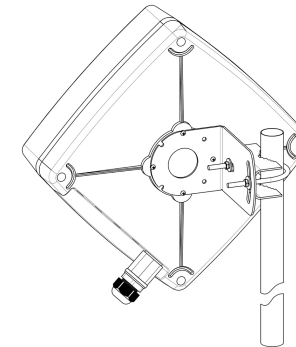
Рисунок 3 – X-поляризация
