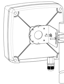
Рисунок 2 – Монтаж антенны
