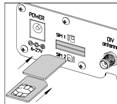
Рисунок 1- Установка SIM-карт
