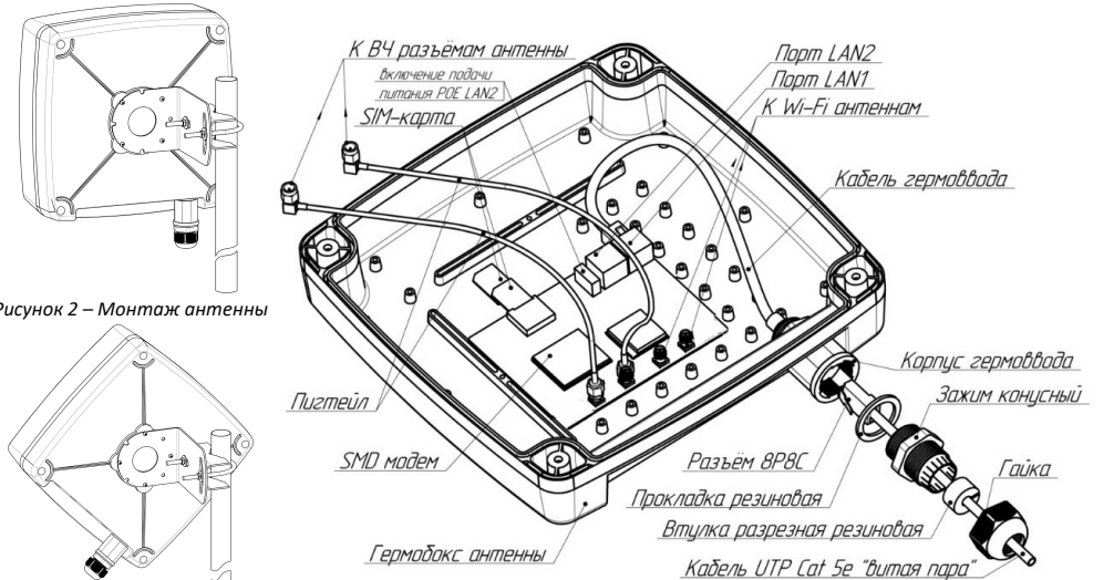
Схема 1 – Размещение роутера в гермобоксе антенны и его подключение
