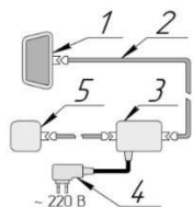
Схема подключения:
