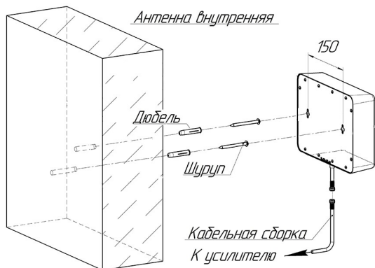
Схема 2 – Монтаж внутренней антенны
