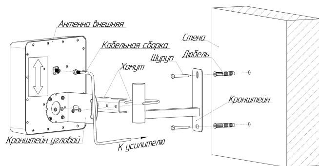
Схема 1 – Монтаж антенны на кронштейн КН-200
