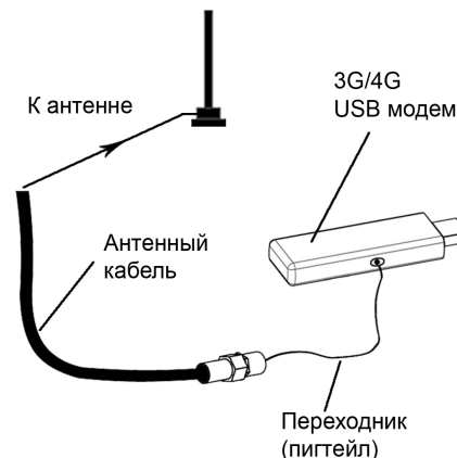
Схема 1 – Подключение антенны к USB модему
