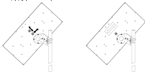
Рисунок 3 – X-поляризация
