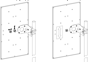
Рисунок 2 – монтаж антенны на мачте
