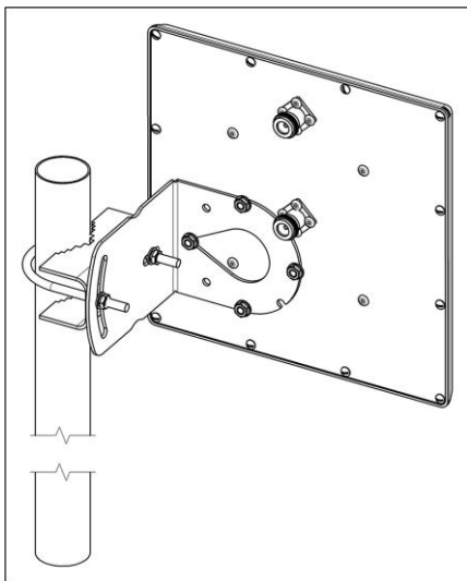
Рисунок 2 – Монтаж антенны на мачте
